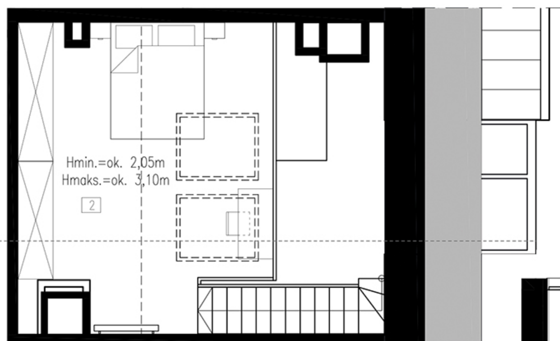
POZIOM +I
